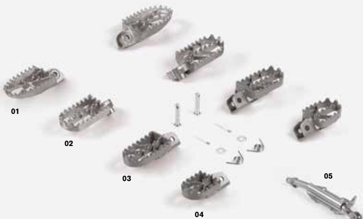
JEU DE REPOSE-PIED FOOT PEGS SET
