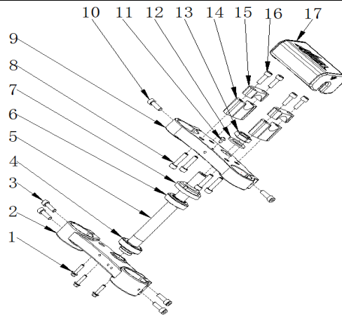
方向把/方向柱 HANDLE BAR/STEERING STEM
