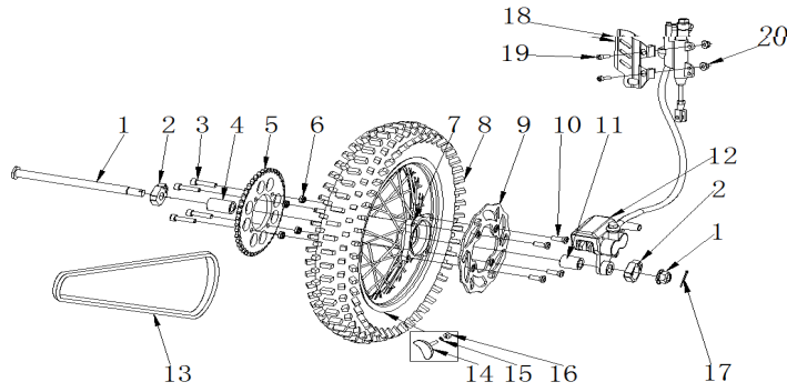
后轮/后制动器 RR.WHEEL/RR. BRAKE ASSY.
